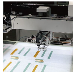
机械手 Manipulator 全自动抓取胶带装置 Automatic tape grabbing device
