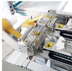
胶带库 Tape library 全自动剪胶带装置 Automatic tape cutting device
