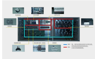
电控柜内部走线强弱分离、所有电气件符合UL认证标准
