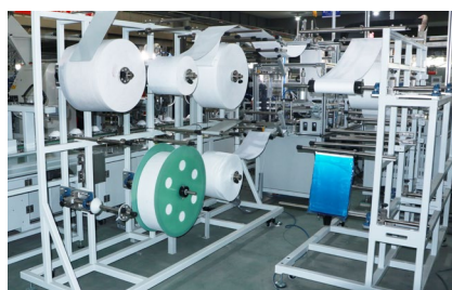
料架
