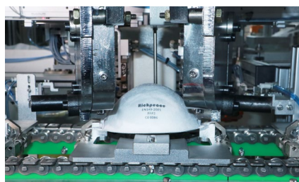
头带打钉
