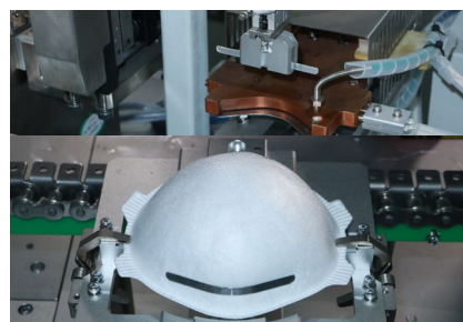
鼻梁条焊接
