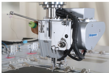
旋转机头 (高速运动件DLC镀膜增加寿命)
