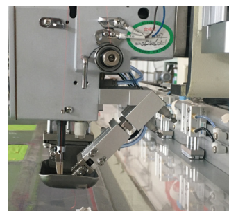
后置上夹线装置
