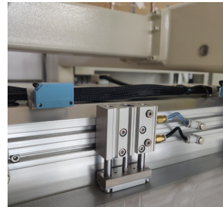
模板到位识别功能
