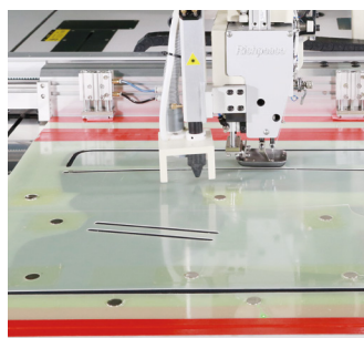
激光切割装置
