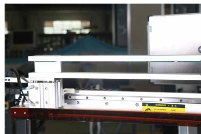
进口SMC气动部件配合料夹，将切断后的材料整理到料箱边沿，方便拾取
