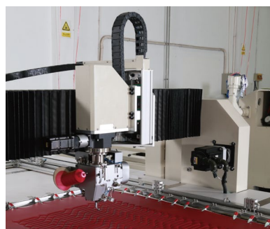
升降式旋转皮革缝纫机头
