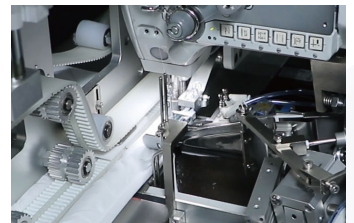
自动收尾装置，使被子缝制完成 收尾处对齐，更加精准美观
