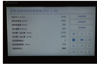
富怡自主研发电控系统
