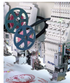
双亮片装置
