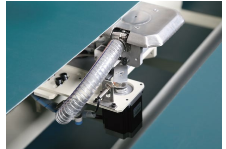
【剪线装置】 上表面无线头，大幅降低底线损耗
