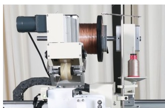
自动送线装置
