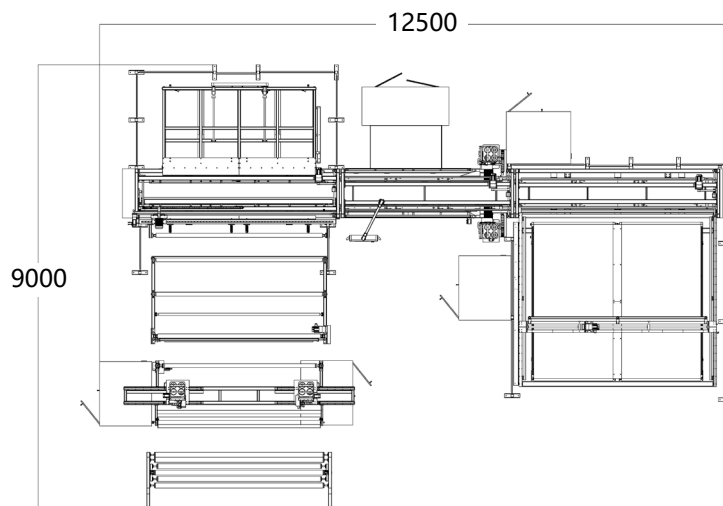
纵缝机头
