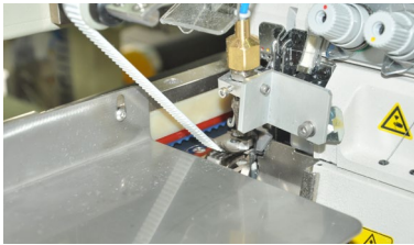
横缝机头
