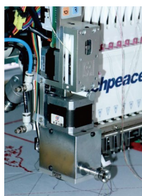
跟踪绳绣装置
