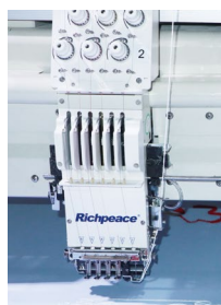
简易绳绣装置
