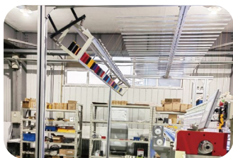
独立面线架及穿线装置
