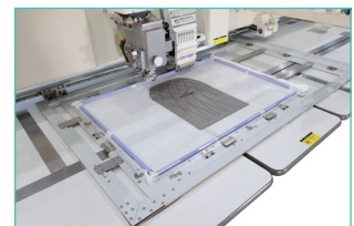
专用工装 Special Fixture
