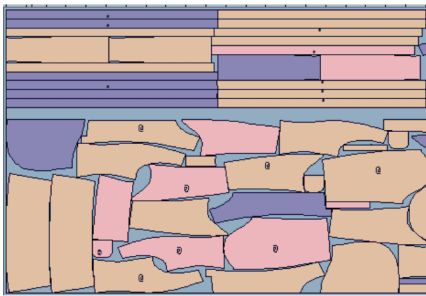
避瑕疵排料 Blemish Avoidance Nest
