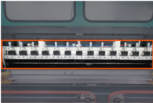
后扫装置 Rear Sweeping Towels
