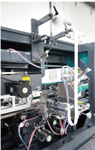
上标机构 Automatic Labelling
