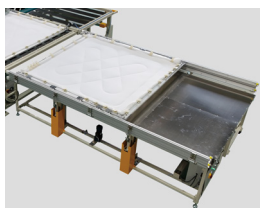
伸缩式自动上料台 (选配) Automatic frame changer (Optional)
