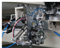
自动换梭 (选配) Automatic bobbin changer (Optional)
